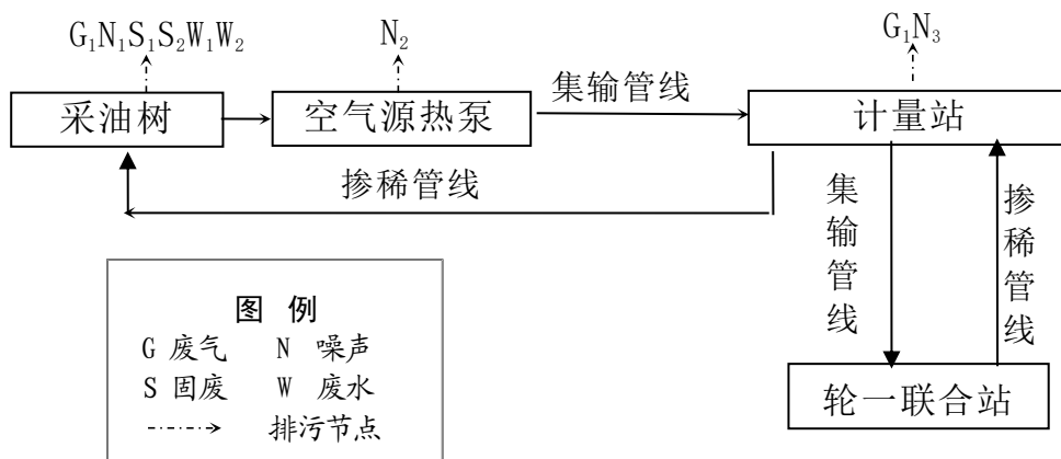
图 3.3-4 井场油气开采及集输工艺流程图
