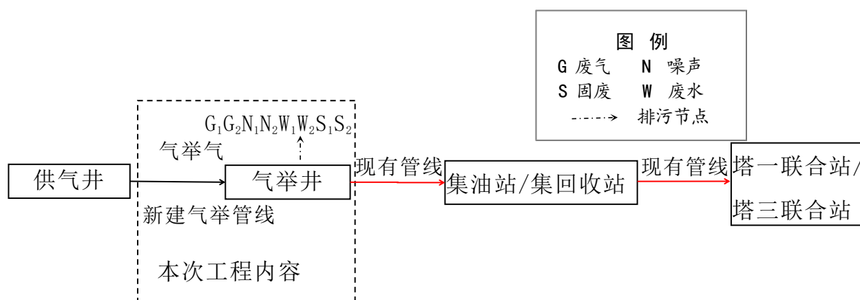
图 3.3-2 井场油气开采及集输工艺流程图
