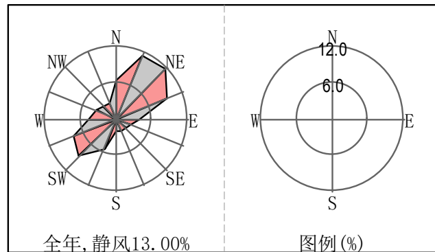
图 5.2-1 近 20 年风频玫瑰图
