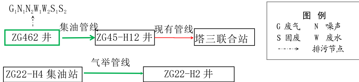
图 3.3-2 井场油气开采及集输工艺流程图
