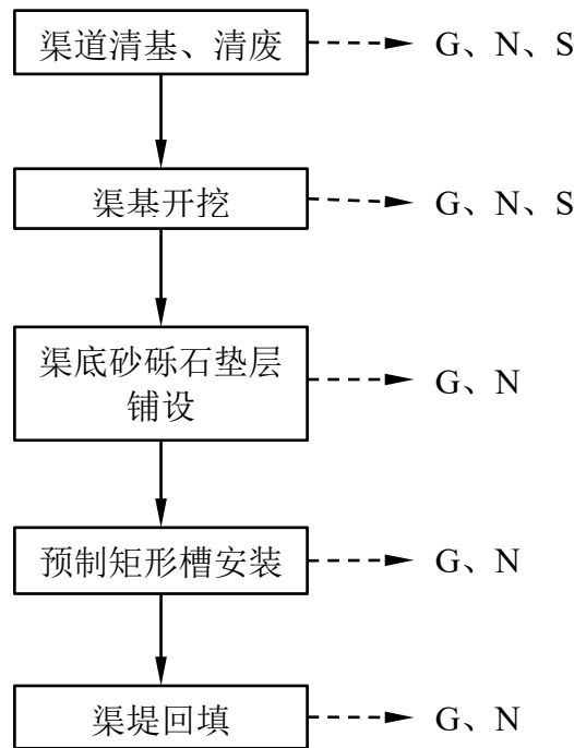
图 3.3-1 施工期渠道施工工艺流程及产污节点图
