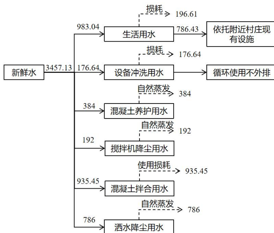
图 3.2-5 项目整个施工期水量平衡示意图 单位: m³
