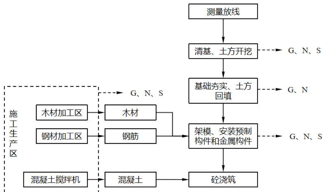
图 3.3-2 施工期渠系建筑物施工工艺流程及产污节点图
