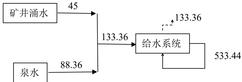
图 3.3-1 运营期水平衡图 单位: \text{m}^3/\text{d}
