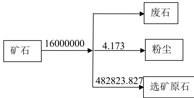
图 3.4-1 物料平衡图 单位: t/a
