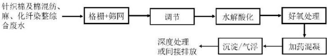
图 7.3-7 针织棉及棉混纺、麻、化纤染整综合废水常规处理工艺流程图
