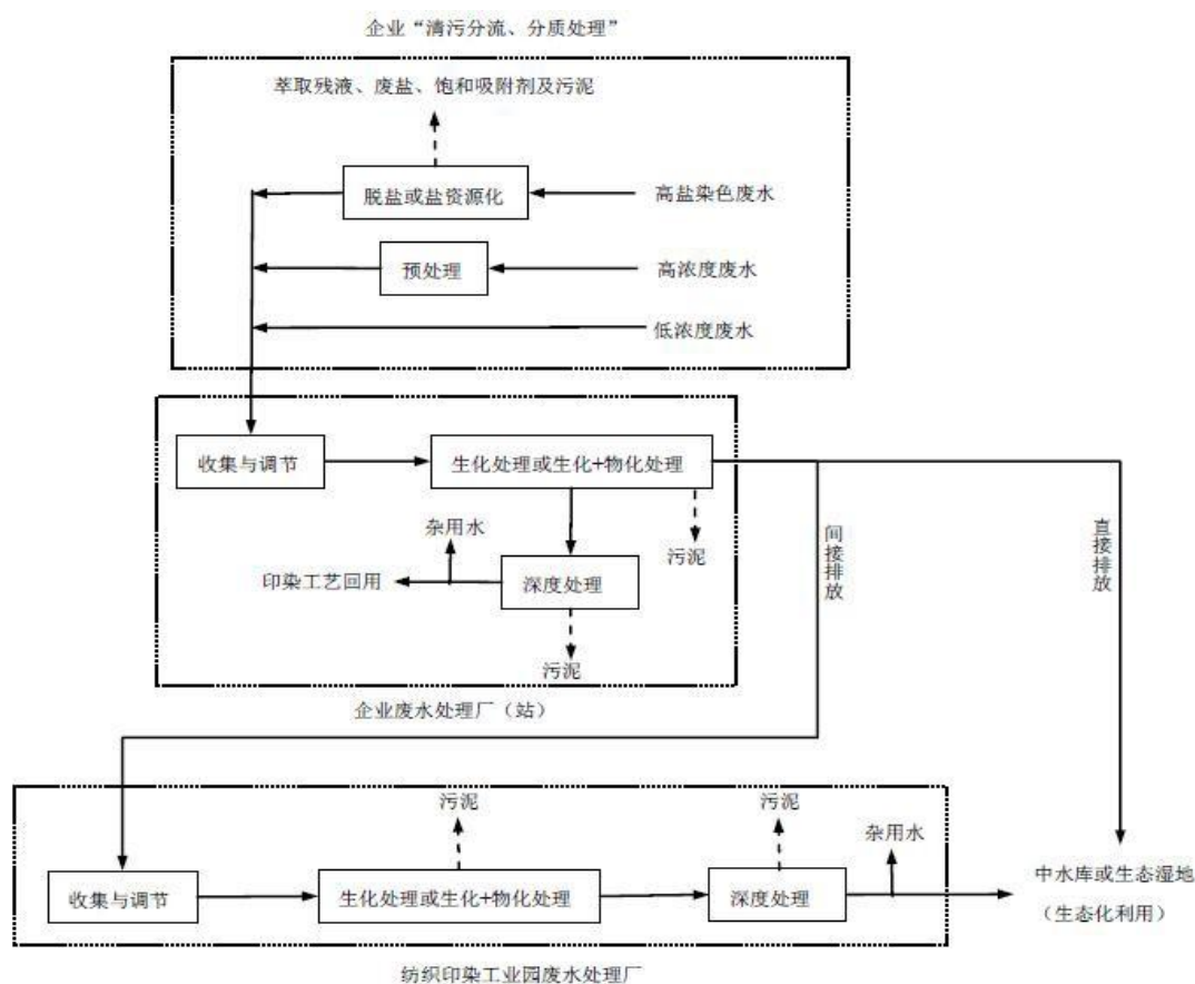
图 7.3-7 印染废水治理全流程示意图
