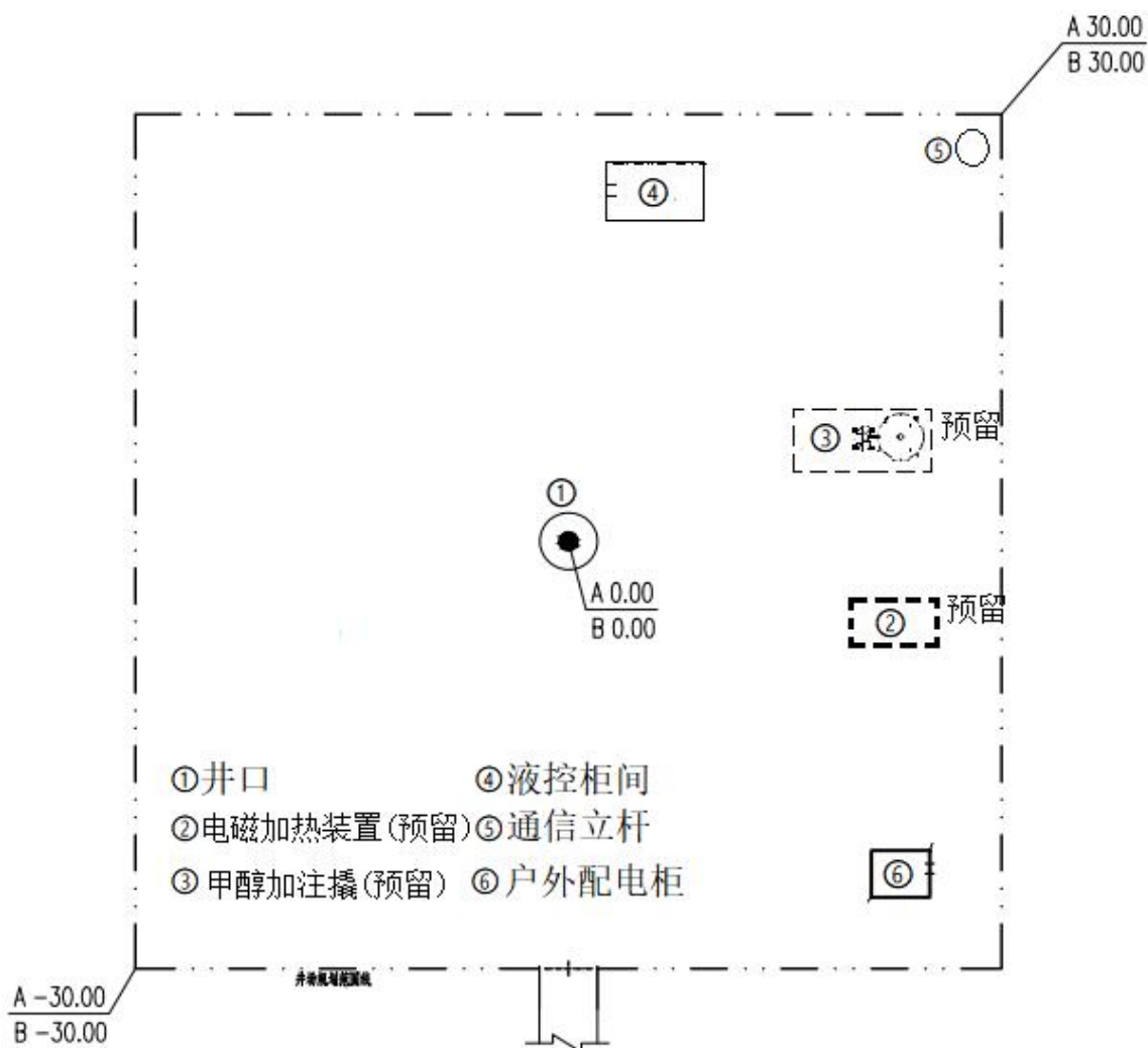
图 3.2-4 新建井场平面布置示意图
