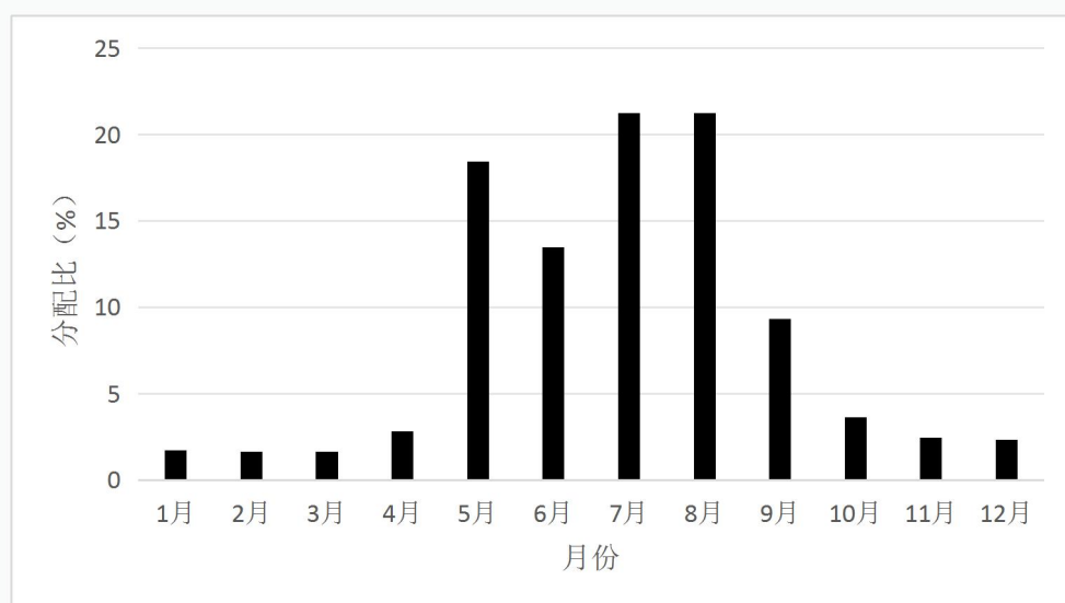
图 6.2-1 东黑沟渠首处年径流量月分配图
