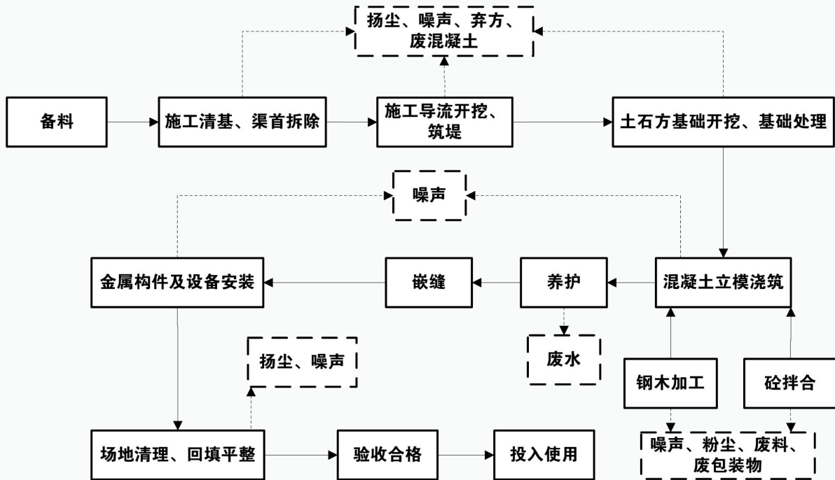
图 4.5-1 主体工程施工流程及产污环节图
