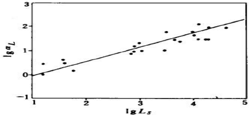
图 5.2-6 \alpha_L — L_s 关系图
