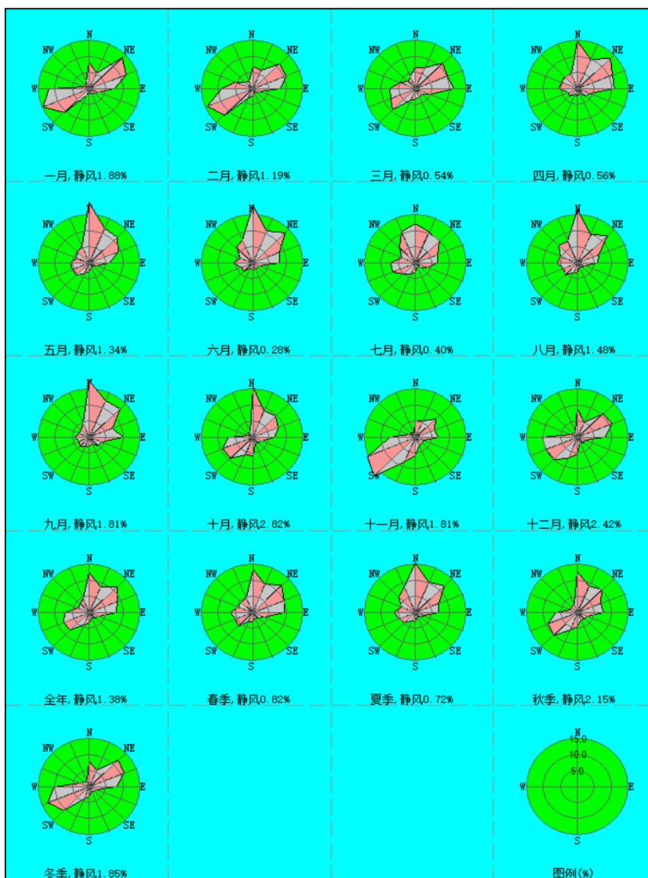
图 5.2-3 年各月、各季及全年风向玫瑰图
