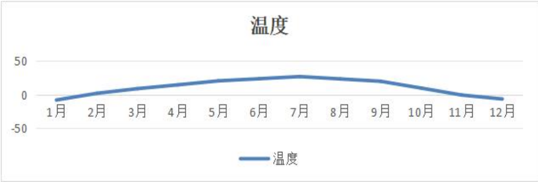
图 5.2-1 年各月平均气温月变化曲线图
