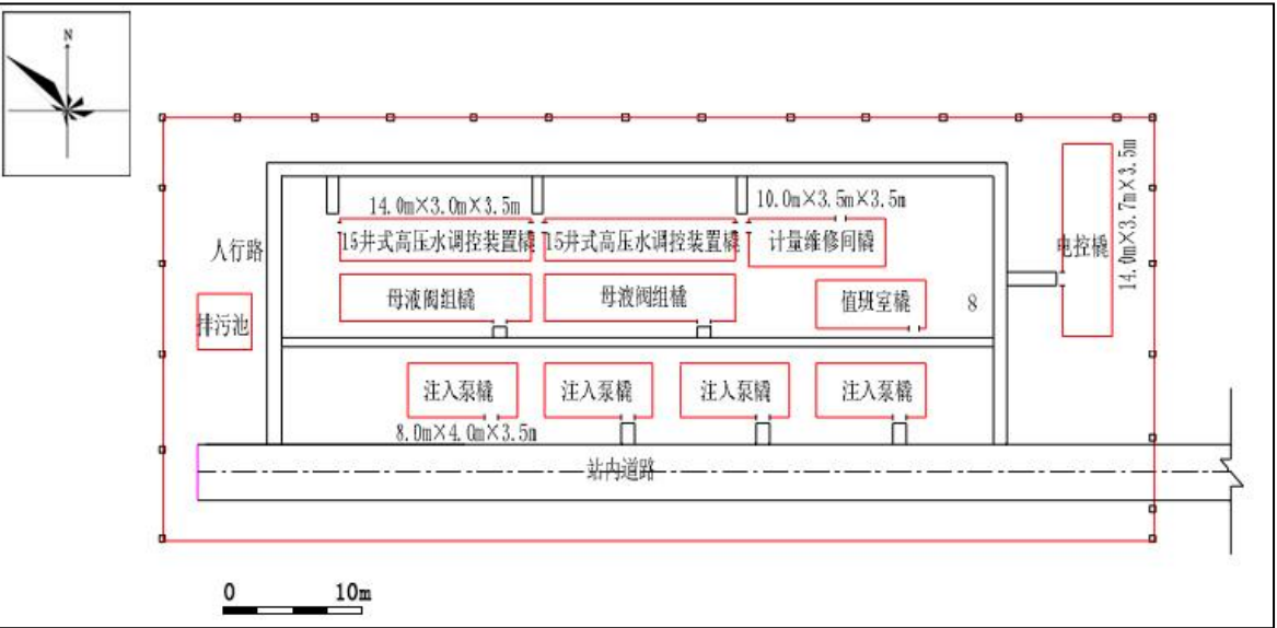
图3.4-4 新建注入站平面布置示意图
