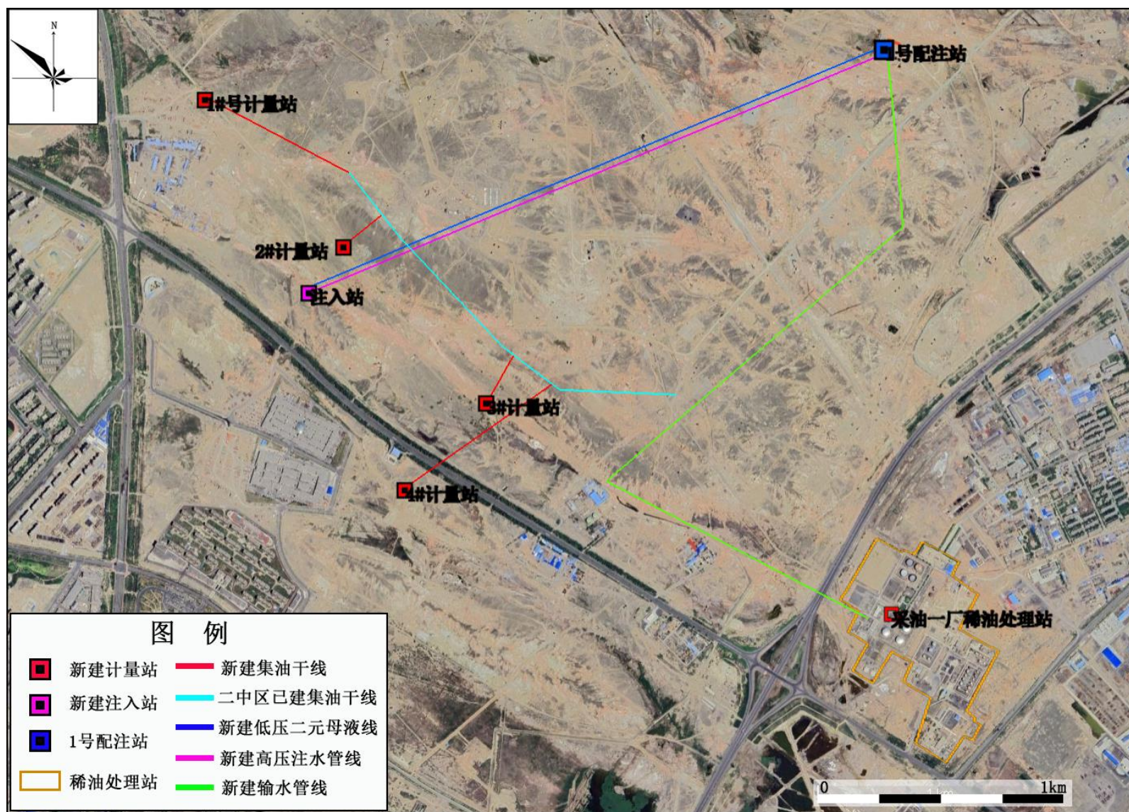
图3.4-6 项目主体工程总平面布置图
