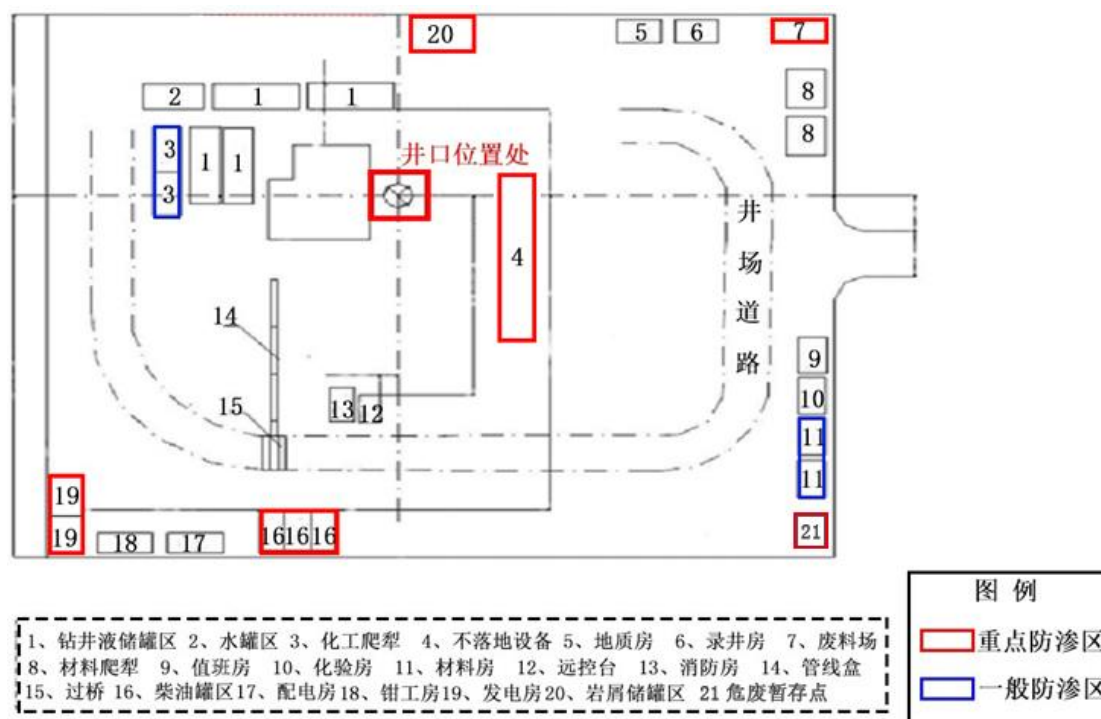
图3.4-3 钻井期井场平面布置示意图
