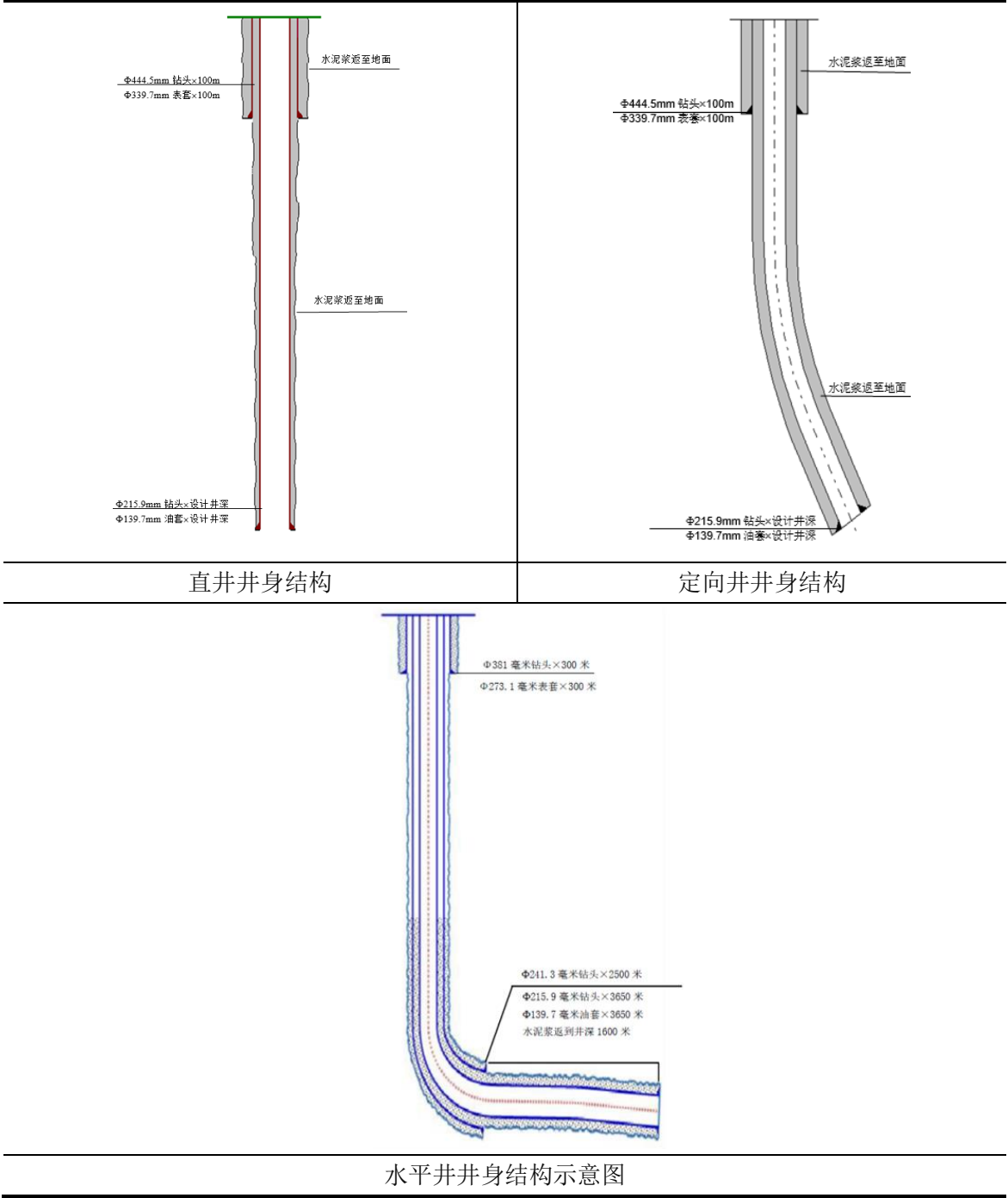
图3. 4-2 井身结构示意图
