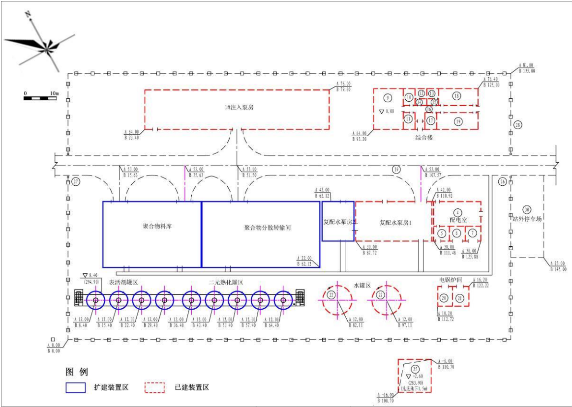
图3.4-5 扩建后配注站平面布置示意图
