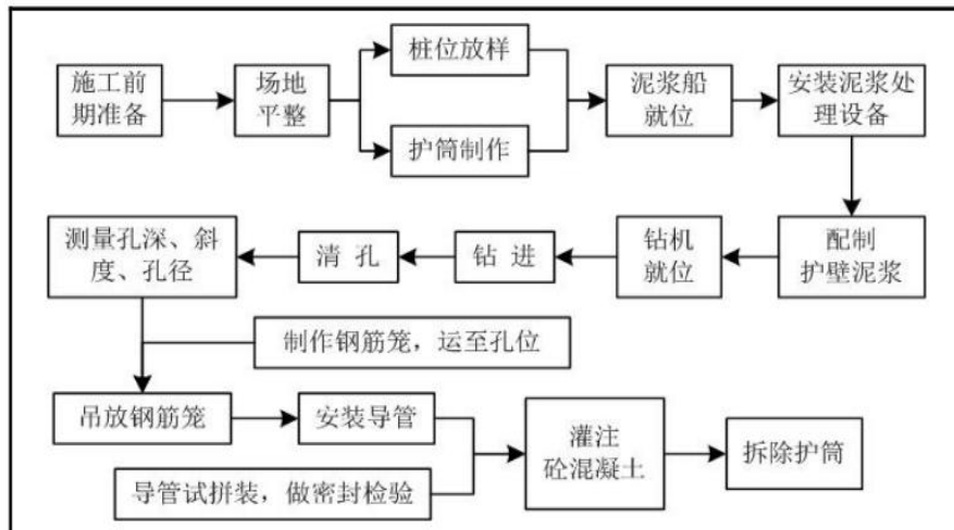
图 3.5-3 钻孔灌注桩基础施工工艺流程图
