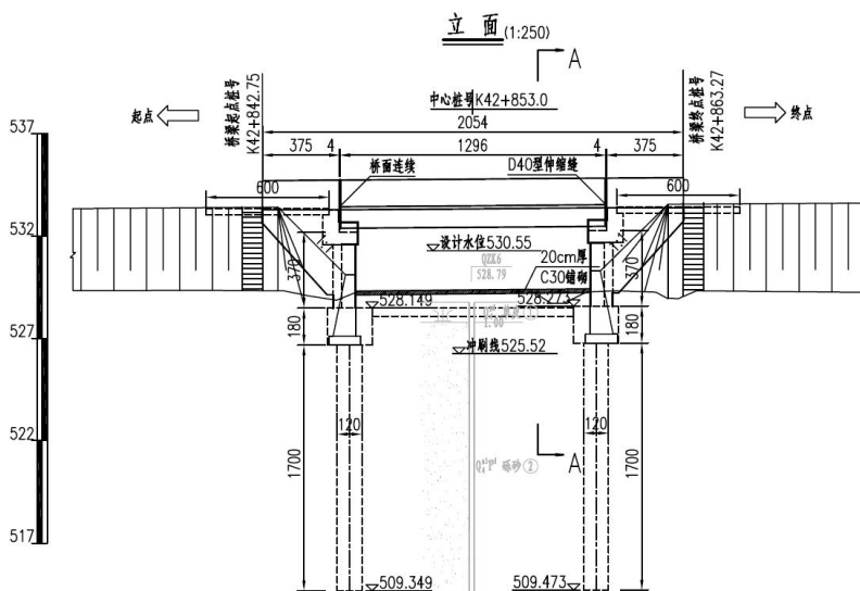
图 3.3-13 小桥设计立面示意图 (K42+853.0)
