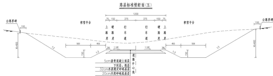
图 3.3-5 本项目路基横断面示意图（五）
