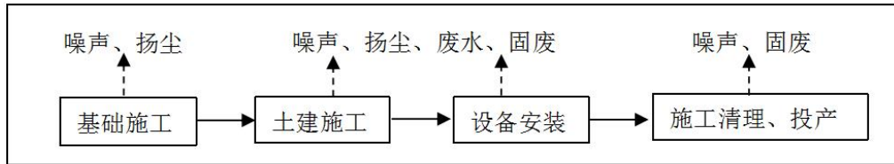
图 3.5-2 养护站施工期工艺及产污环节图
