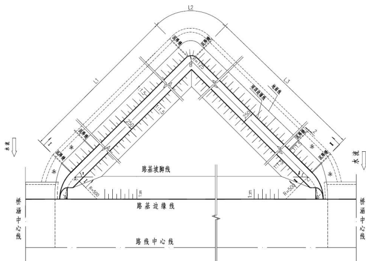
图 3.3-9 本项目导流坝设计示意图 (II 型)
