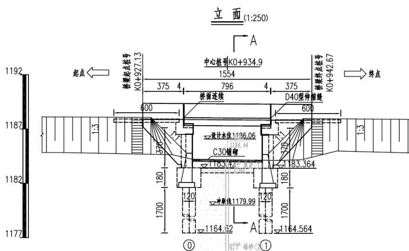
图 3.3-11 小桥设计立面示意图 (K0+934.9)
