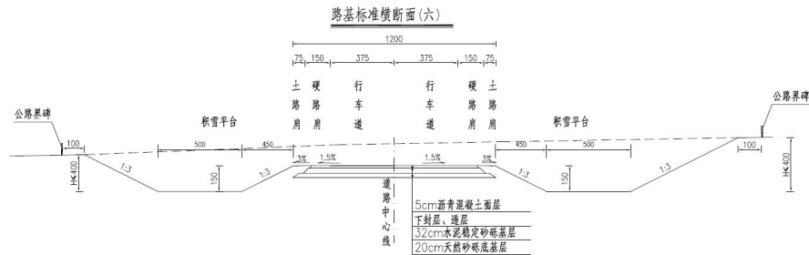
图 3.3-6 本项目路基横断面示意图（六）
