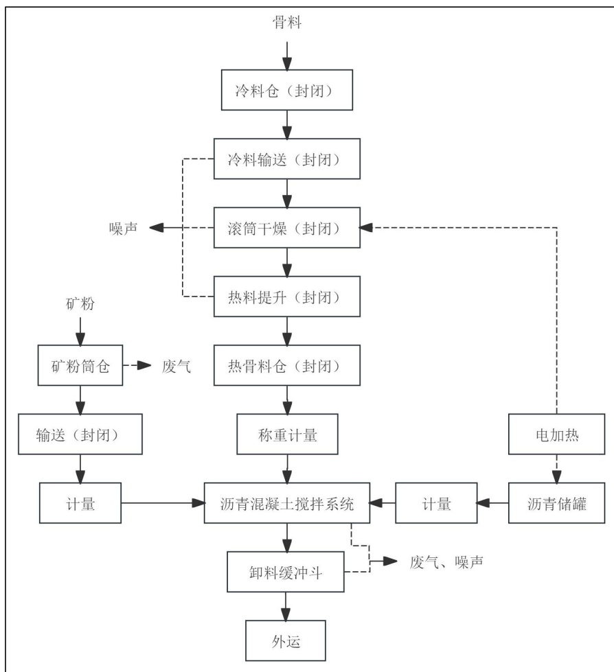
图 3.5-5 沥青混凝土拌合工艺流程示意图
