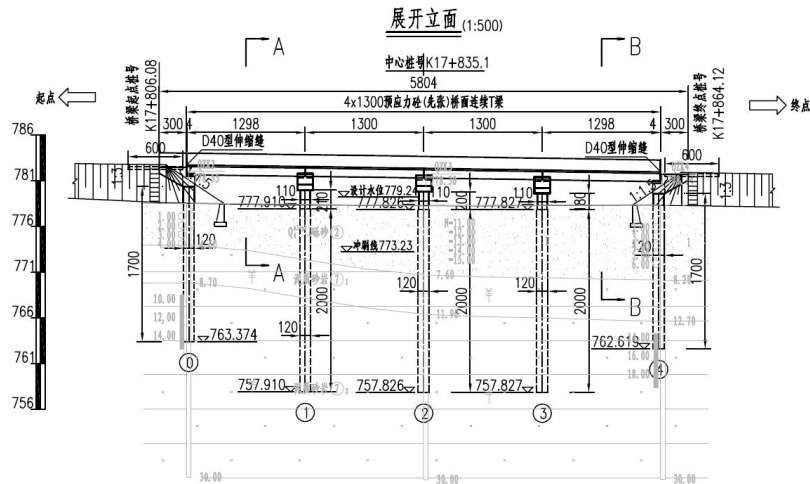
图 3.3-10 中桥设计立面示意图 (K17+835.1)
