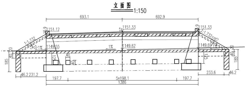
图 3.3-18 本项目典型涵洞设计示意图（以 K2+372.3 为例）
