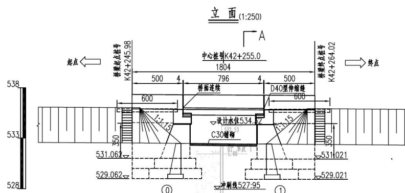
图 3.3-12 小桥设计立面示意图 (K42+255)
