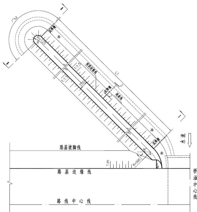
图 3.3-8 本项目导流坝设计示意图 (I 型)
